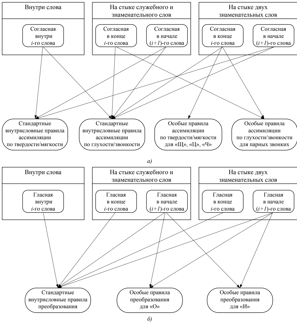
Рис. Особенности внутрисловных и межсловных правил преобразования буква-фонема: а) для согласных; б) для гласных
